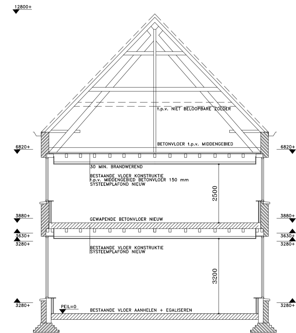
DOORSNEDE
